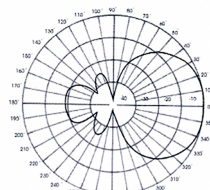
Diagramme de rayonnement vertical
