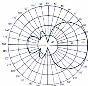
Diagramme de rayonnement vertical
