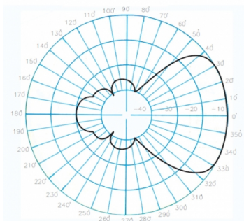
Diagramme de rayonnement horizontal
