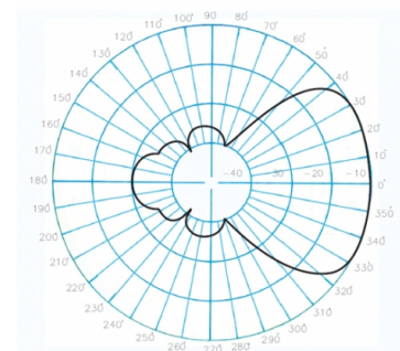
Diagramme de rayonnement horizontal
