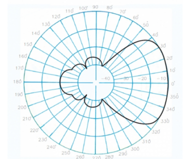
Diagramme de rayonnement horizontal
