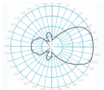
Diagramme de rayonnement vertical
