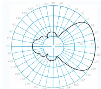
Diagramme de rayonnement vertical. Diagramme de rayonnement horizontal sans préavis
