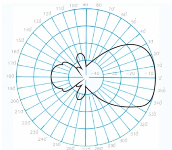
Diagramme de rayonnement vertical. Diagramme de rayonnement horizontal sans préavis
